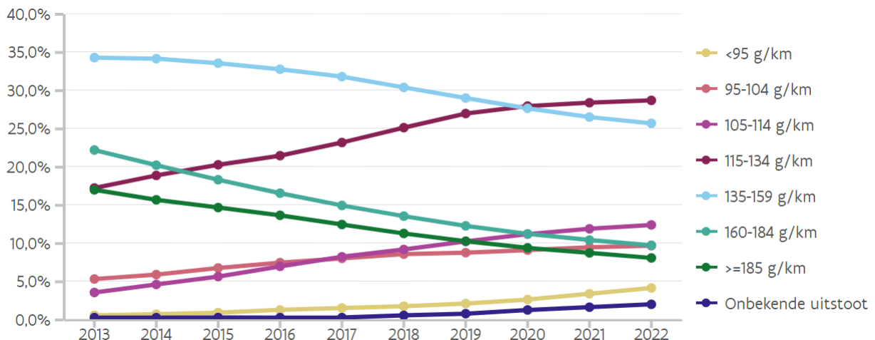
Milieuvriendelijkheid van het wagenpark naar CO 2 -uitstoot, 2013-2022, in procenten (Aalst)
